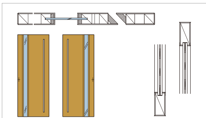
Fスリット (シングル)
