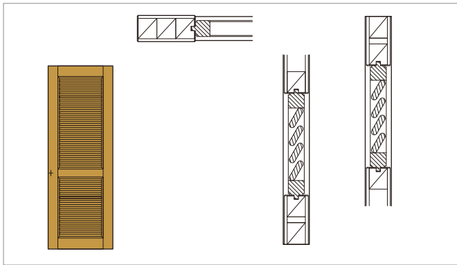
ガラリ付建具(片流れ)
