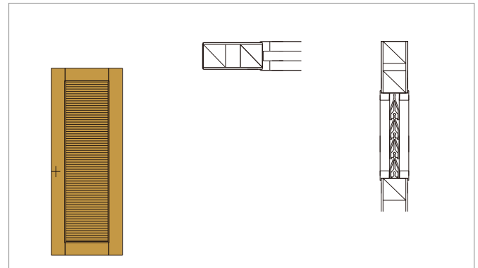
ガラリ付建具(山型)
