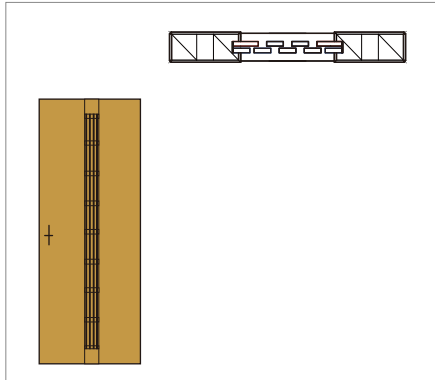
IVスリット (112型)
